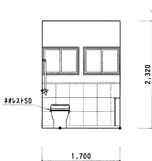
B面展開図 1/50
