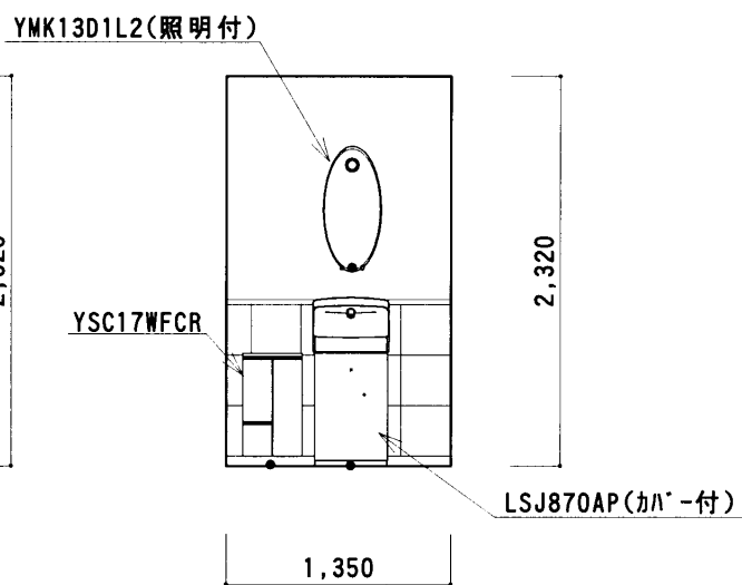
C面展開図 1/50
