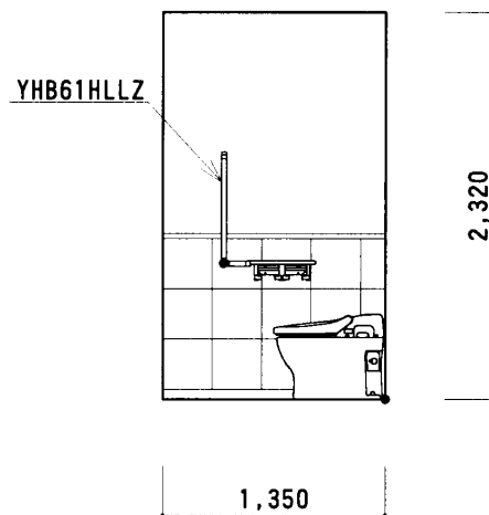
A面展開図 1/50
