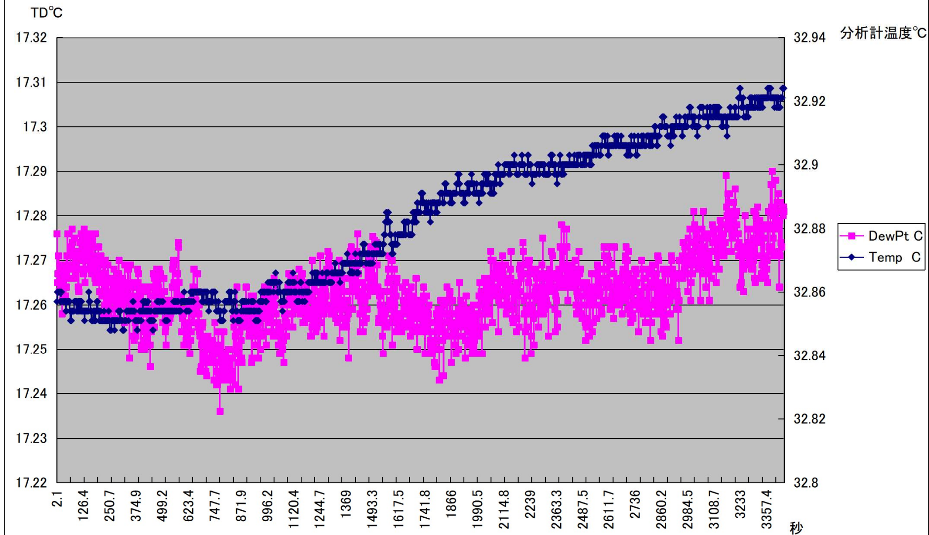
DP75-E露点制御通気ユニット設定17.3TD°CでのLI-6262分析計での長時間測定約50分
