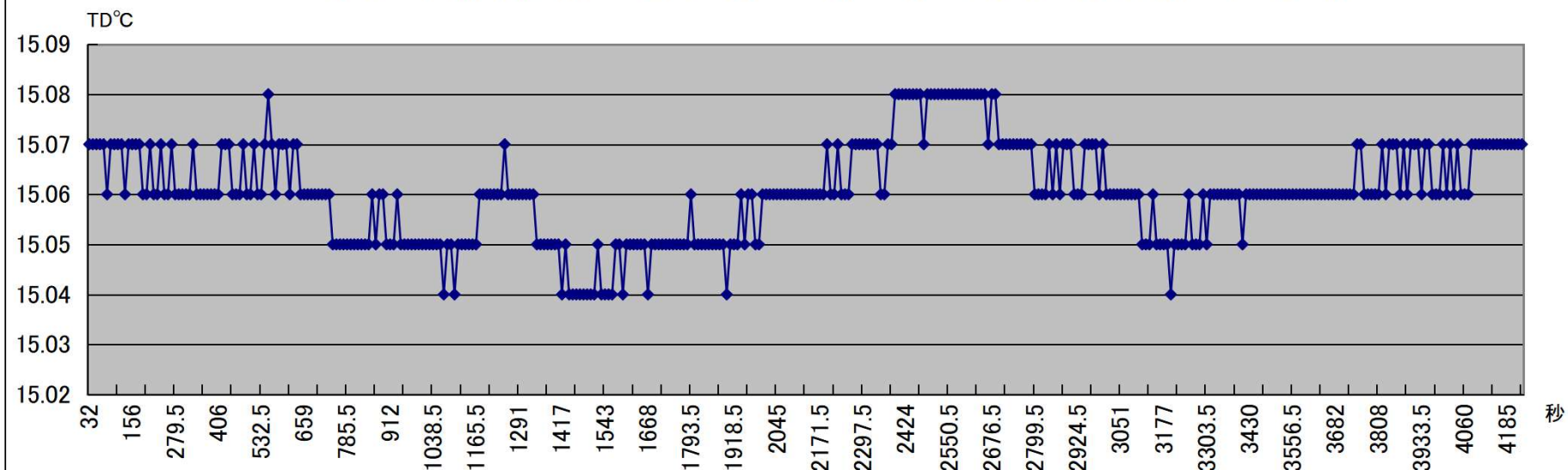
DP75-E 露点制御通気ユニットTD15. 0℃設定時のLI-6400TdSでの実測データ 約1時間
