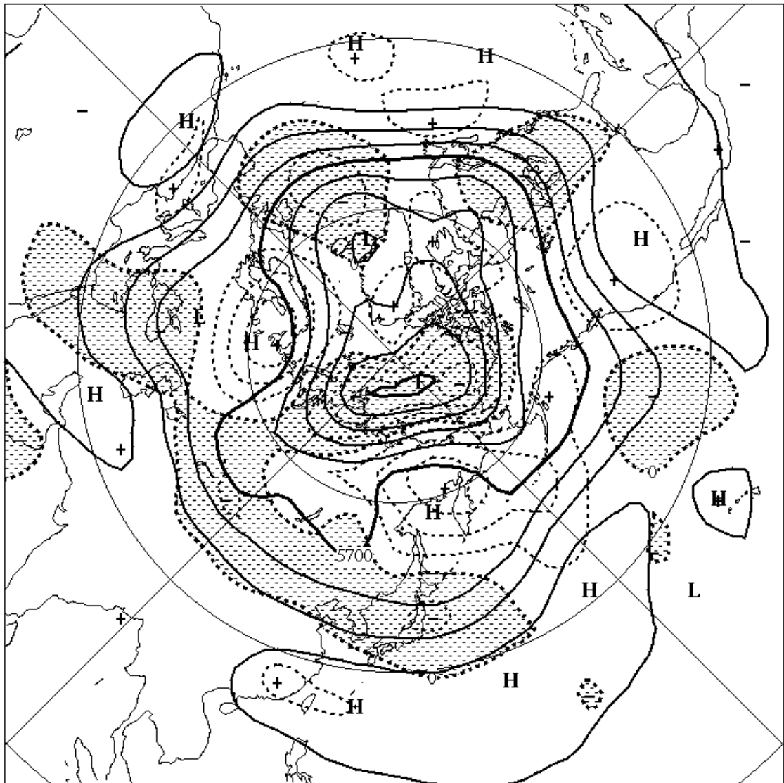
2003 年 7 月の 500hPa 高度・偏差（等値線間隔 実況（実線）60m、偏差（破線）30m） 陰影域は負偏差
