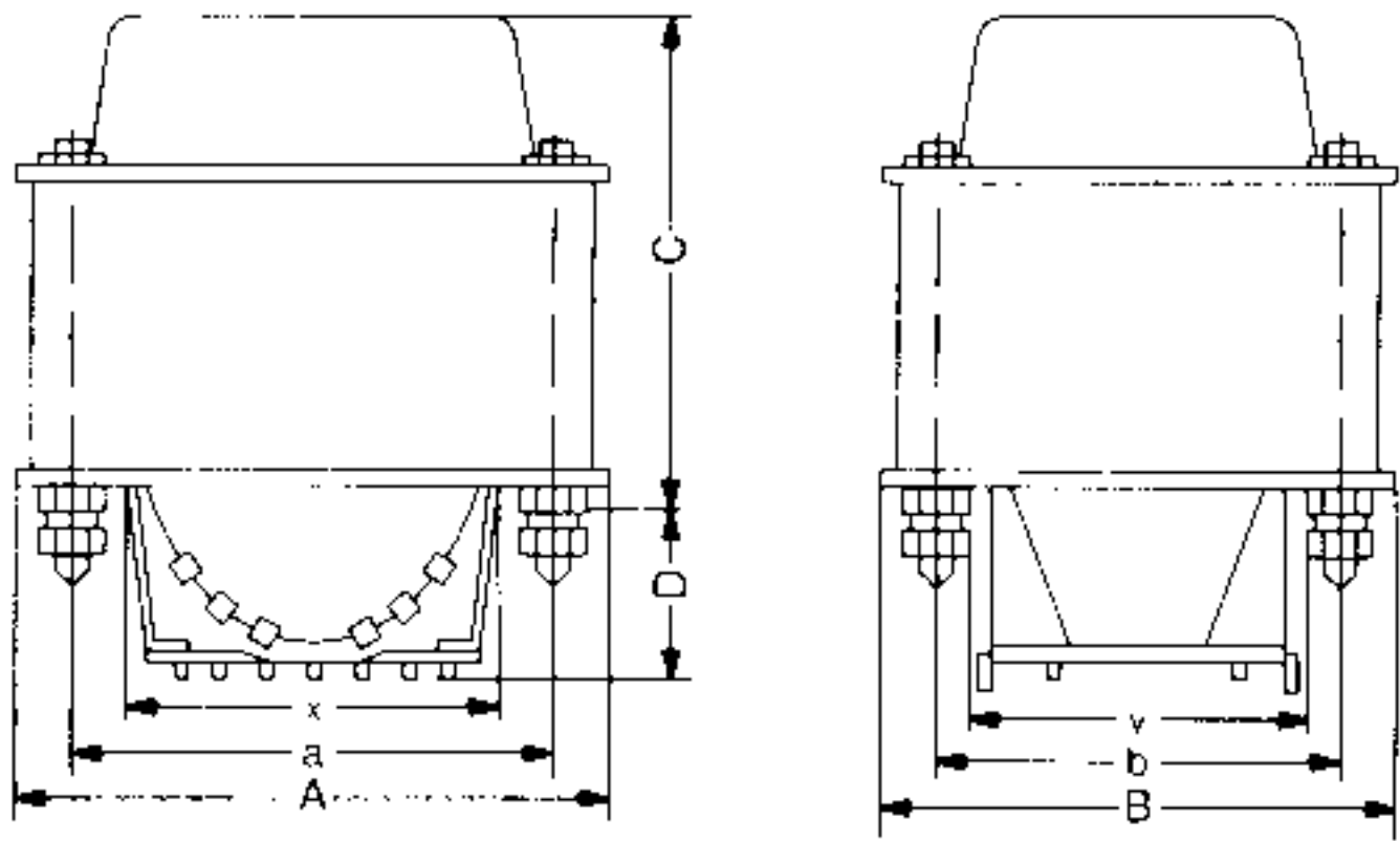
端子板式及び伏型ラグ
