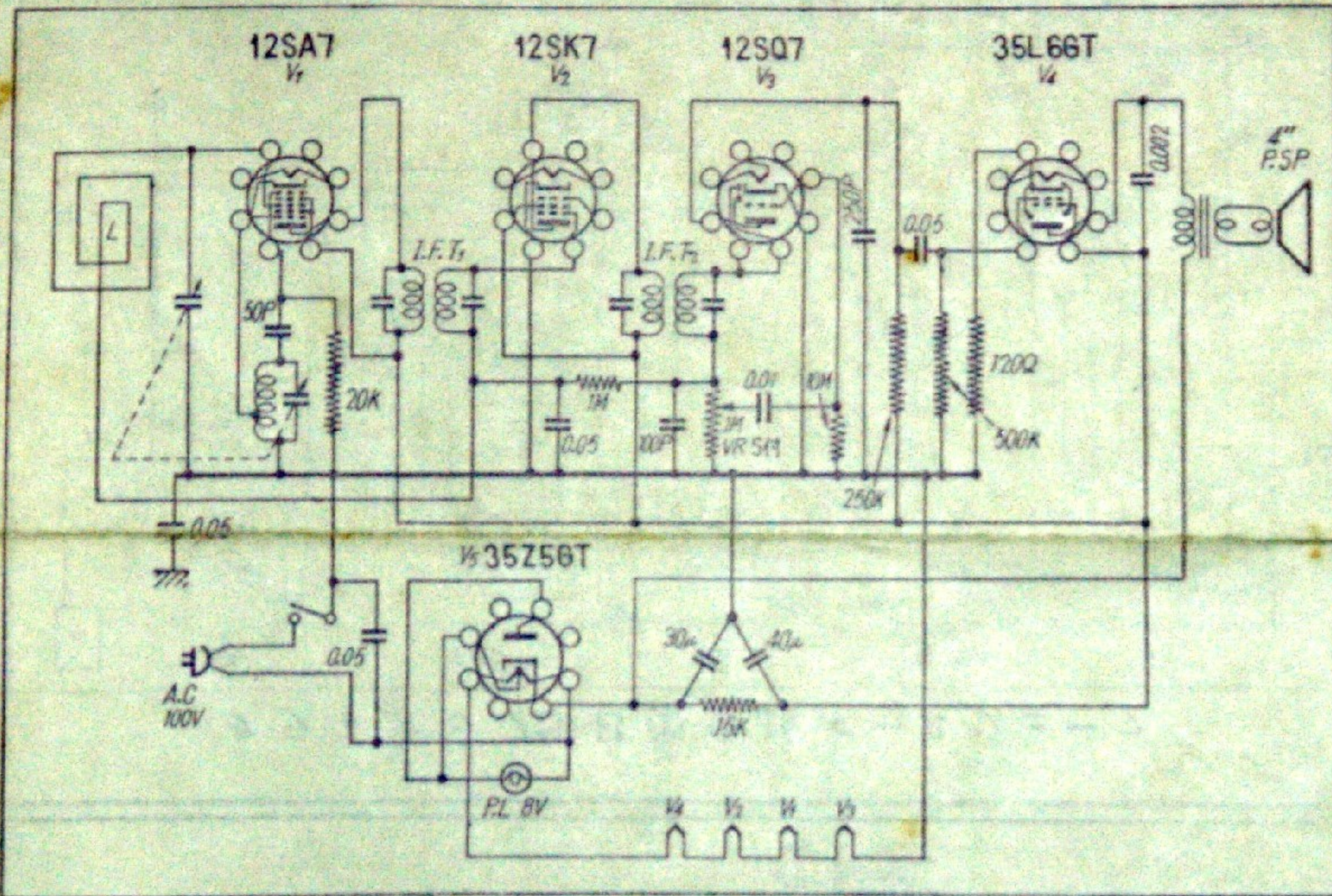
NRC A-21型 トランスレス5球スーパー
