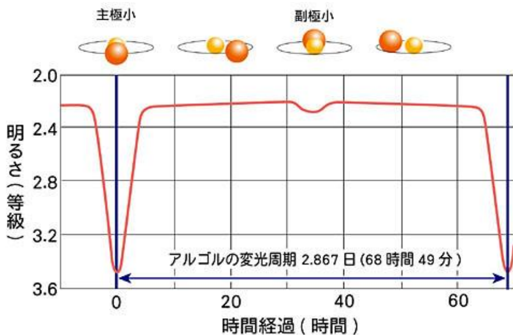
食変光星「アルゴルの光度変化」
