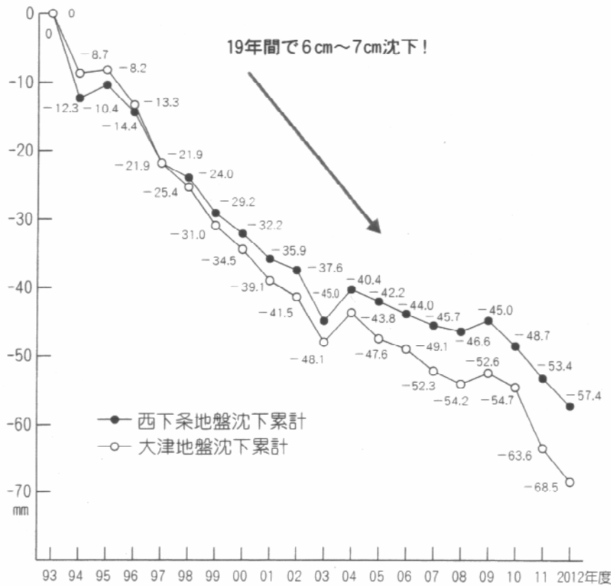
『南部工業団地地盤沈下測量結果』甲府市商工課資料より作成
