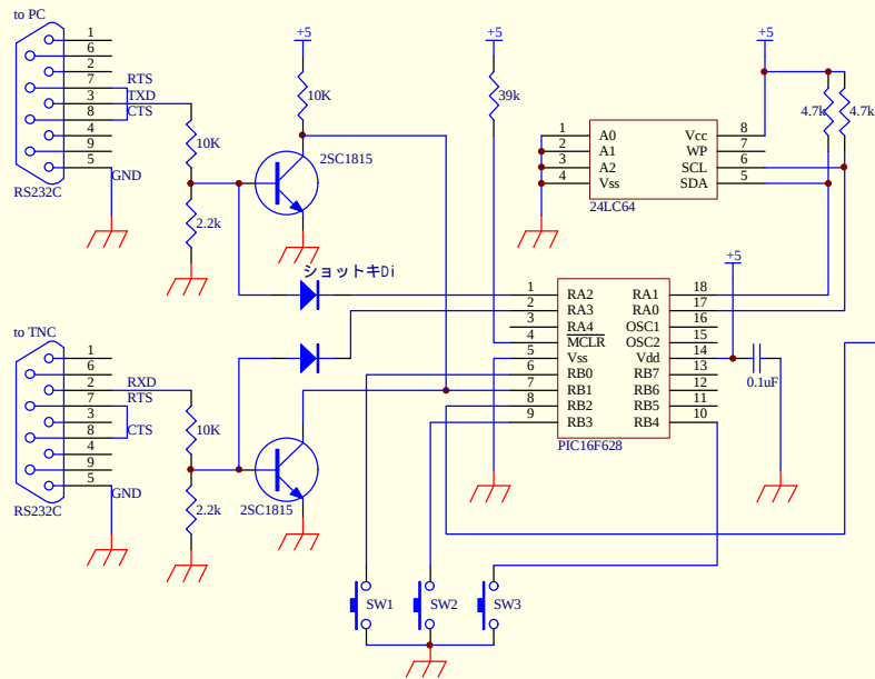
回路図 * 5
