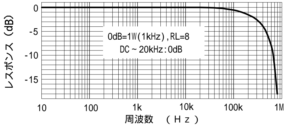
図 18 周波数特性
