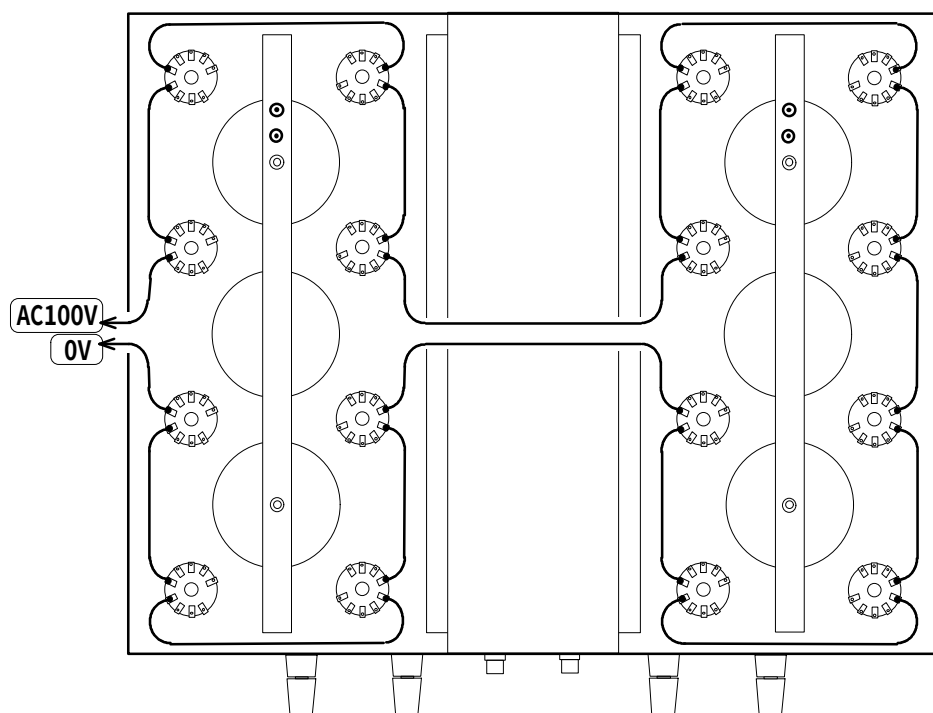
図 12 ヒーターの配線
