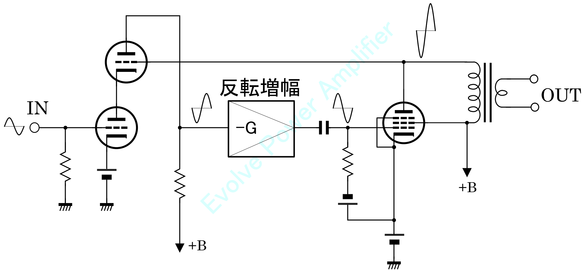
[ 図2 ] 超3結Vの基本回路
