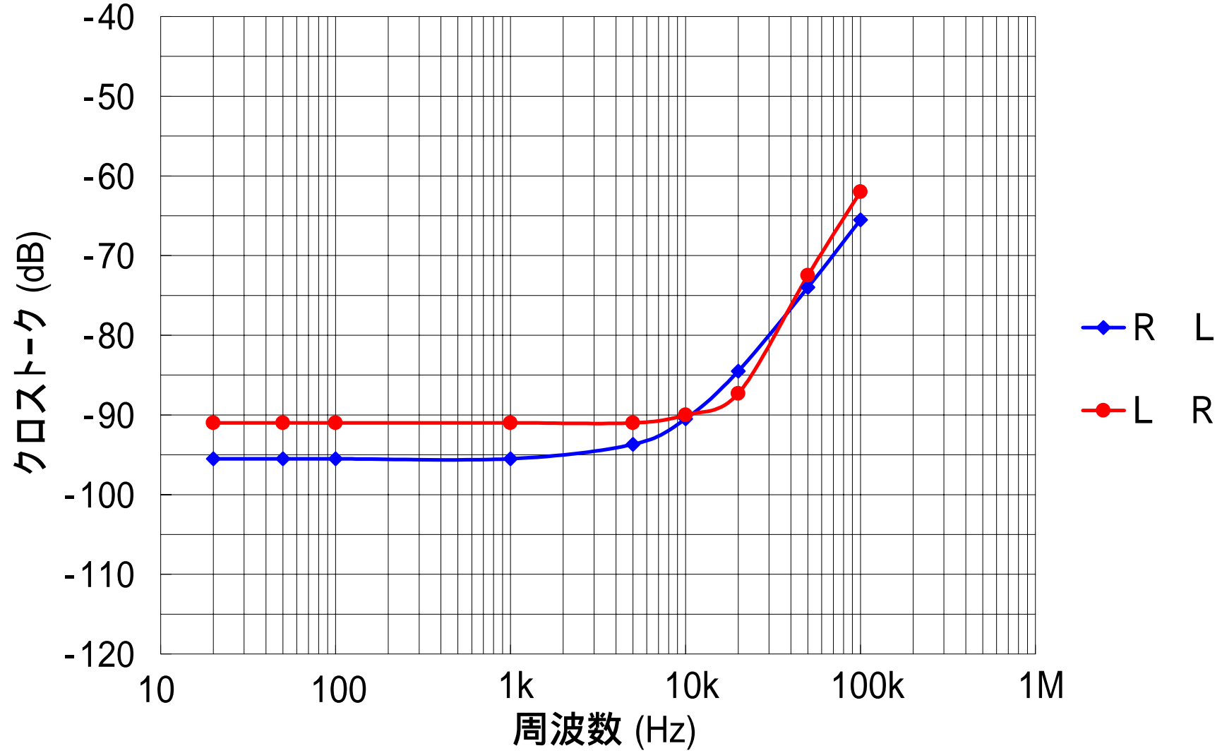
[ 図15 ] クロストーク特性
