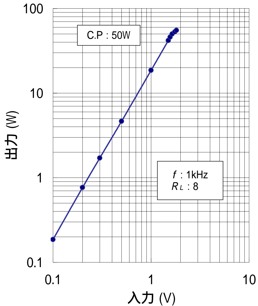
[ 図11 ] 入出力特性
