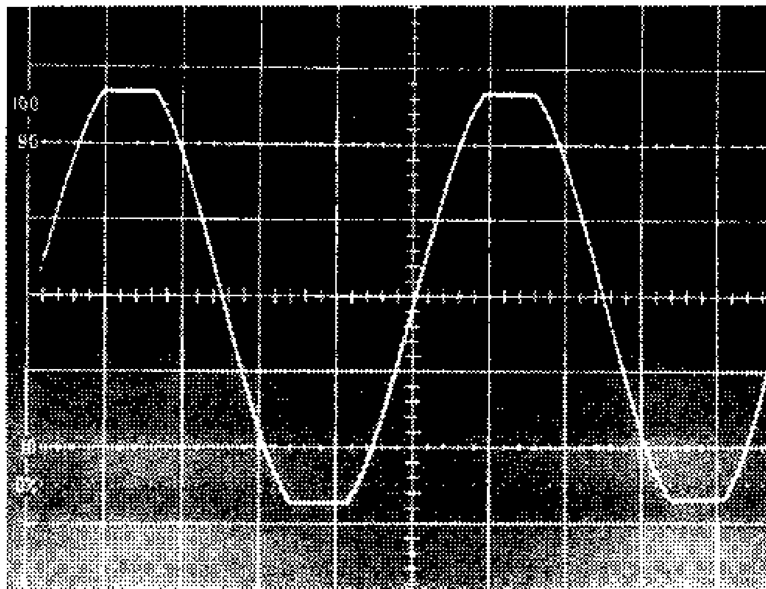
[写真1] 10kHz クリップ波形. V軸: 10V/DIV. 負荷: 8Ω
