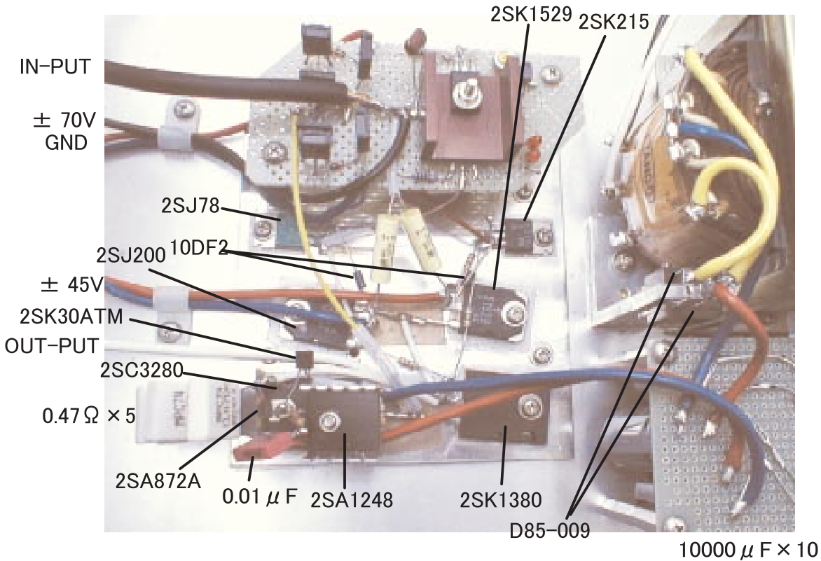
[ 写真1 ] アンプ部分の配線
