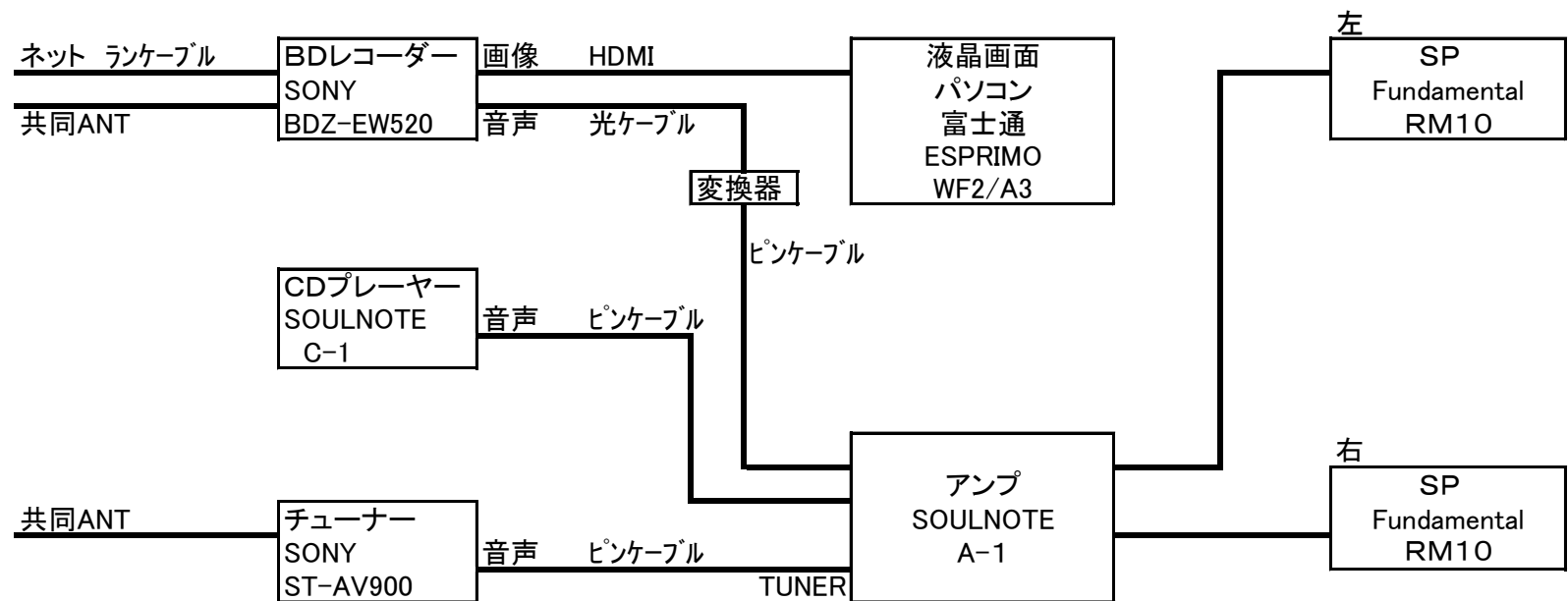
AV機器接続概要図 2017.6.5記
