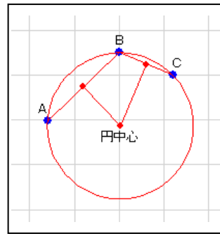
円の中心は、線分A-Bと、線分B-Cの midpoint からの垂線を算出し、2つの垂線の交点であることを示します。尚、円の半径は、円中心から3点(A, B, C)のいずれかまでの長さとなります。
